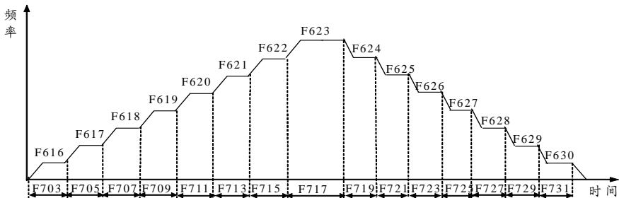
图 6-24 程序运行
